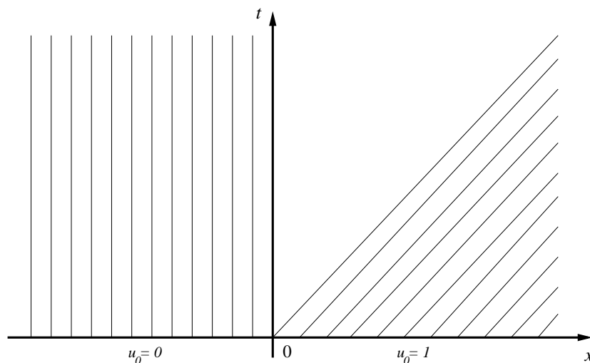
Figura 18.8: Curvas características planares para a equação de Burgers inviscível com a condição inicial u_0 = 0 para x \leq 0 e u_0 = 1 para x > 0 . Acima, exibimos apenas o semiplano t \geq 0 . As retas do lado esquerdo são verticais e as do lado direito têm inclinação 1. Observe que as curvas características planares não visitam a região t \geq x com x > 0 . Esse fenômeno é relacionado às chamadas ondas de rarefação da Mecânica dos Fluidos.
