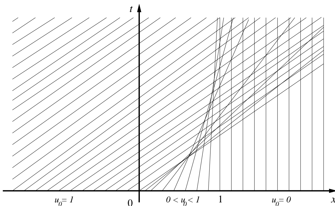
Figura 18.6: As curvas características planares no semiplano t \geq 0 associadas à condição inicial u_0 de (18.83). As retas que partem do eixo x na região x \leq 0 correspondem a s_2 < 0 e têm inclinação 1. As retas que partem do eixo x na região 0 < x < 1 correspondem a 0 < s_2 < 1 e têm inclinação variando de 1 a infinito. As retas que partem do eixo x na região x \geq 1 correspondem a s_2 \geq 1 e têm inclinação infinita, ou seja, são verticais. A função u é constante ao longo de cada curva característica planar, assumindo em cada uma o valor fixado pela função u_0 no ponto onde mesma atinge o eixo horizontal x (i.e., em t = 0 ). Porém, em pontos em que ocorrem cruzamentos de curvas características planares, há uma indefinição. Observe na figura acima a existência de zonas de cruzamento das curvas características planares. Essas zonas são regiões singulares onde ocorrem as chamadas ondas de choque .
