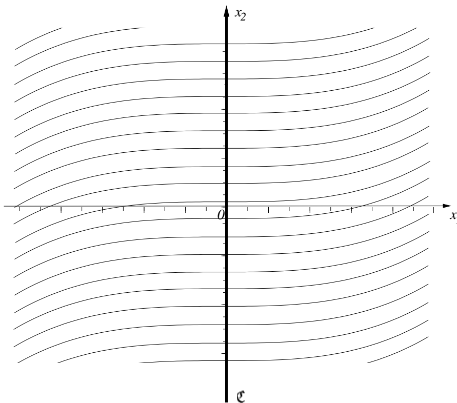
Figura 18.2: Curvas características planares da equação (18.66) no plano x_1-x_2 . A superfície de Cauchy \mathfrak{C} é eixo vertical x_2 .
