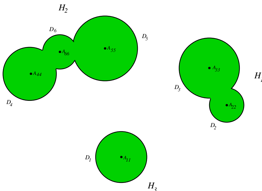
Figura 10.1: No plano complexo, os discos de Gershgorin D_1, \dots, D_6 de uma matriz A complexa 6 \times 6 e as correspondentes regiões conexas H_1 = D_2 \cup D_3 , H_2 = D_4 \cup D_5 \cup D_6 e H_3 = D_1 . Os centros dos discos são os elementos diagonais da matriz: A_{11}, \dots, A_{66} e seus raios são as grandezas \varrho_1, \dots, \varrho_6 . Neste exemplo, h_1 = 2 , h_2 = 3 e h_3 = 1 .
