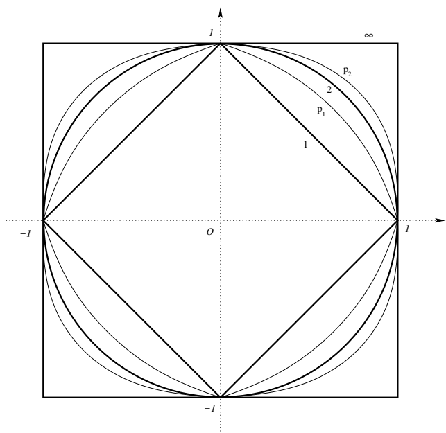
Figura 3.1: As bolas \overline{B_1(0)} , de raio 1 centradas em 0, relacionadas às normas \|\cdot\|_p e \|\cdot\|_\infty em \mathbb{R}^2 . As linhas sólidas indicam os bordos \partial B_1(0) . O índice 1 indica a bola \overline{B_1(0)} para a norma \|\cdot\|_1 . Trata-se de um quadrado oblíquo com arestas de comprimento \sqrt{2} centrado na origem O . O índice p_1 indica as bolas \overline{B_1(0)} para as normas \|\cdot\|_{p_1} quando 1 < p_1 < 2 . O índice 2 indica a bola \overline{B_1(0)} para a norma \|\cdot\|_2 . Essa é a única bola que coincide com o disco de raio 1 centrado na origem O . O índice p_2 indica as bolas \overline{B_1(0)} para as normas \|\cdot\|_{p_2} quando p_2 > 2 . O índice \infty indica a bola \overline{B_1(0)} para a norma \|\cdot\|_\infty . Trata-se de um quadrado com arestas de comprimento 2 centrado na origem O .
