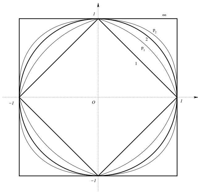
Figura 3.1: As bolas \overline{\mathcal{B}_1(0)} , de raio 1 centradas em 0, relacionadas às normas \|\cdot\|_p e \|\cdot\|_\infty em \mathbb{R}^2 . As linhas sólidas indicam os bordos \partial\mathcal{B}_1(0) . O índice 1 indica a bola \overline{\mathcal{B}_1(0)} para a norma \|\cdot\|_1 . Trata-se de um quadrado obliquo com arestas de comprimento \sqrt{2} centrado na origem O . O índice p_1 indica as bolas \overline{\mathcal{B}_1(0)} para as normas \|\cdot\|_{p_1} quando 1 < p_1 < 2 . O índice 2 indica a bola \overline{\mathcal{B}_1(0)} para a norma \|\cdot\|_2 . Essa é a única bola que coincide com o disco de raio 1 centrado na origem O . O índice p_2 indica as bolas \overline{\mathcal{B}_1(0)} para as normas \|\cdot\|_{p_2} quando p_2 > 2 . O índice \infty indica a bola \overline{\mathcal{B}_1(0)} para a norma \|\cdot\|_\infty . Trata-se de um quadrado com arestas de comprimento 2 centrado na origem O .
