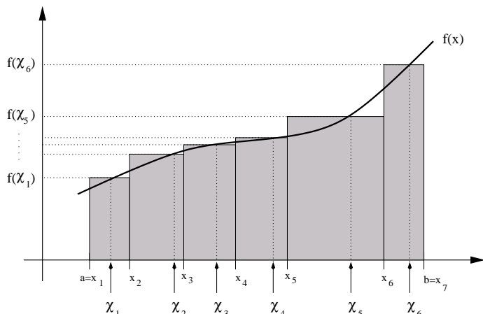
Figura 33.1: Representação da soma de Riemann de uma função f no intervalo [a, b] com a partição \mathcal{P} = \{a = x_1, x_2, x_3, x_4, x_5, x_6, x_7 = b\} , com os pontos intermediários \chi = \{\chi_1, \chi_2, \chi_3, \chi_4, \chi_5, \chi_6\} . O k -ésimo retângulo tem altura f(\chi_k) e largura |I_k| = x_{k+1} - x_k . A soma das áreas desses retângulos fornece S[(\mathcal{P}, \chi), f] .
