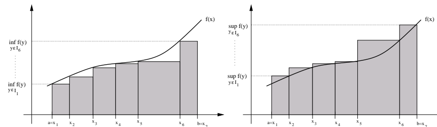
Figura 33.2: Representação das somas de Darboux da mesma função e da mesma partição da Fig. 33.1. A soma das áreas dos retângulos à esquerda fornece D_i[\mathcal{P}, f] e a soma das áreas dos retângulos à direita fornece D_s[\mathcal{P}, f] .
